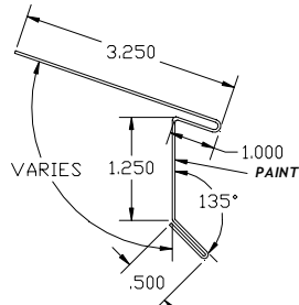
Drip Edge - LDE6
